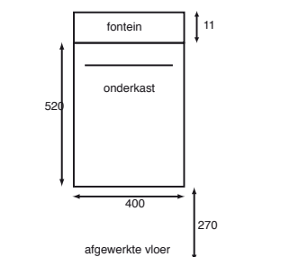
Voor aanzicht 'Excuse Me' fonteinmeubel
