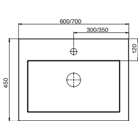
lijntekening gebaseerd op wastafel met 1 kraangat en 1 afvoer
