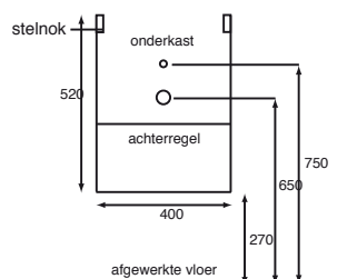
Achteraanzicht onderkast 'Excuse Me' fonteinmeubel
