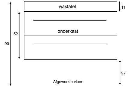
Achteraanzicht onderkast 'Fit Me' 60/70/100 cm (in centimeters)
