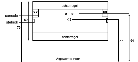
Achteraanzicht onderkast 'Fit Me' 60/70/100 cm (in centimeters)
