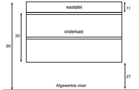
Achteraanzicht onderkast 'Touch Me' 60/70/100 cm (in centimeters)
