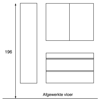
Vooraanzicht 'Touch Me' 60/70/100/120cm (in centimeters)
