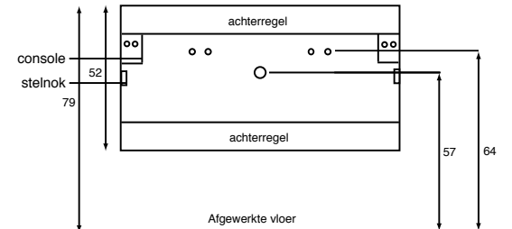
Achteraanzicht onderkast 'Fit Me' 100 cm (in centimeters)
