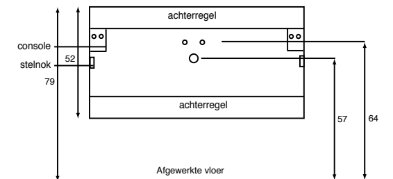
Achteraanzicht onderkast 'Touch Me' 60/70/100 cm (in centimeters)
