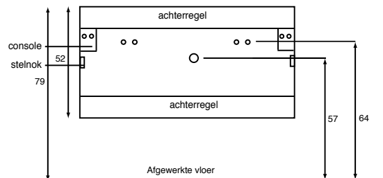
Achteraanzicht onderkast 'Touch Me' 100 cm (in centimeters)
