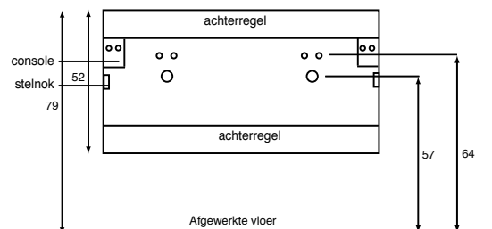
Achteraanzicht onderkast 'Touch Me' 120 cm (in centimeters)
