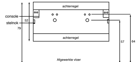
Achteraanzicht onderkast 'Fit Me' 120 cm (in centimeters)
