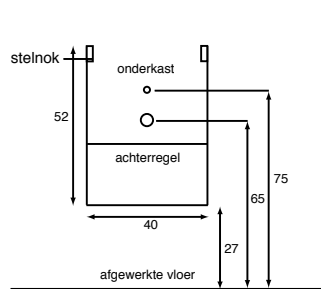
Achteraanzicht onderkast 'Excuse Me' fonteinmeubel (in centimeters)
