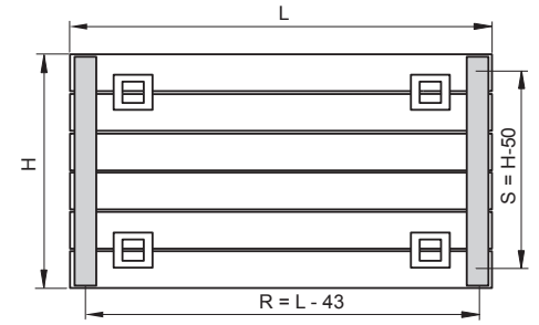
Achteraanzicht / Vista trasera
