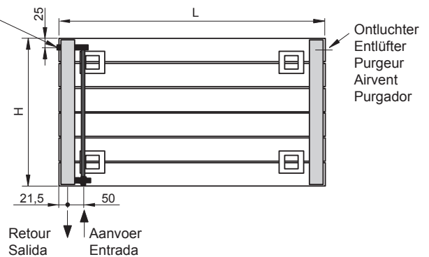
Ventieladiator / Radiator con válvula integrada
