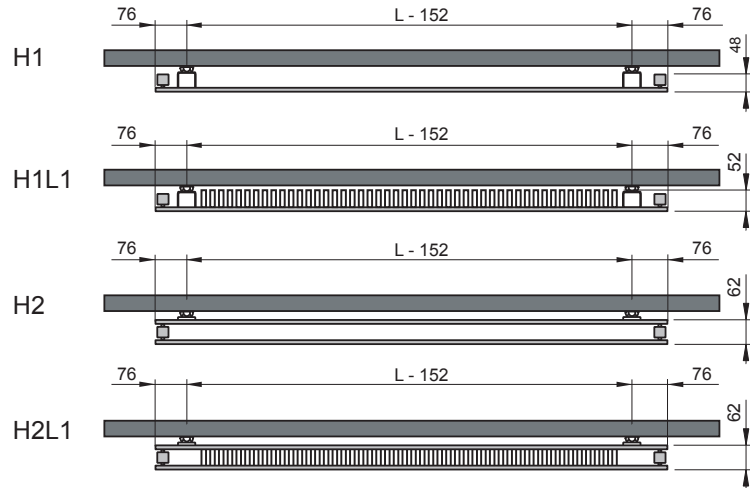
Bovenaanzicht / Vista por arriba
