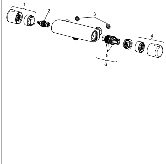
Producttekening
