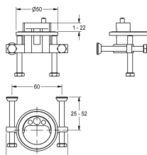
DOORDRAAIBEVEILIGING
