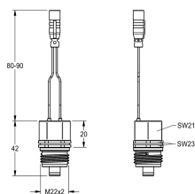
PATROON VOORZIEN VAN MAGNEETKLEP
