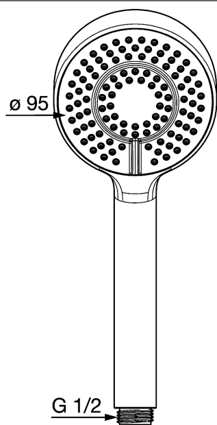
Producttekening
