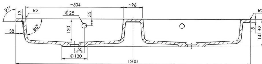
B-B (1 : 5)
