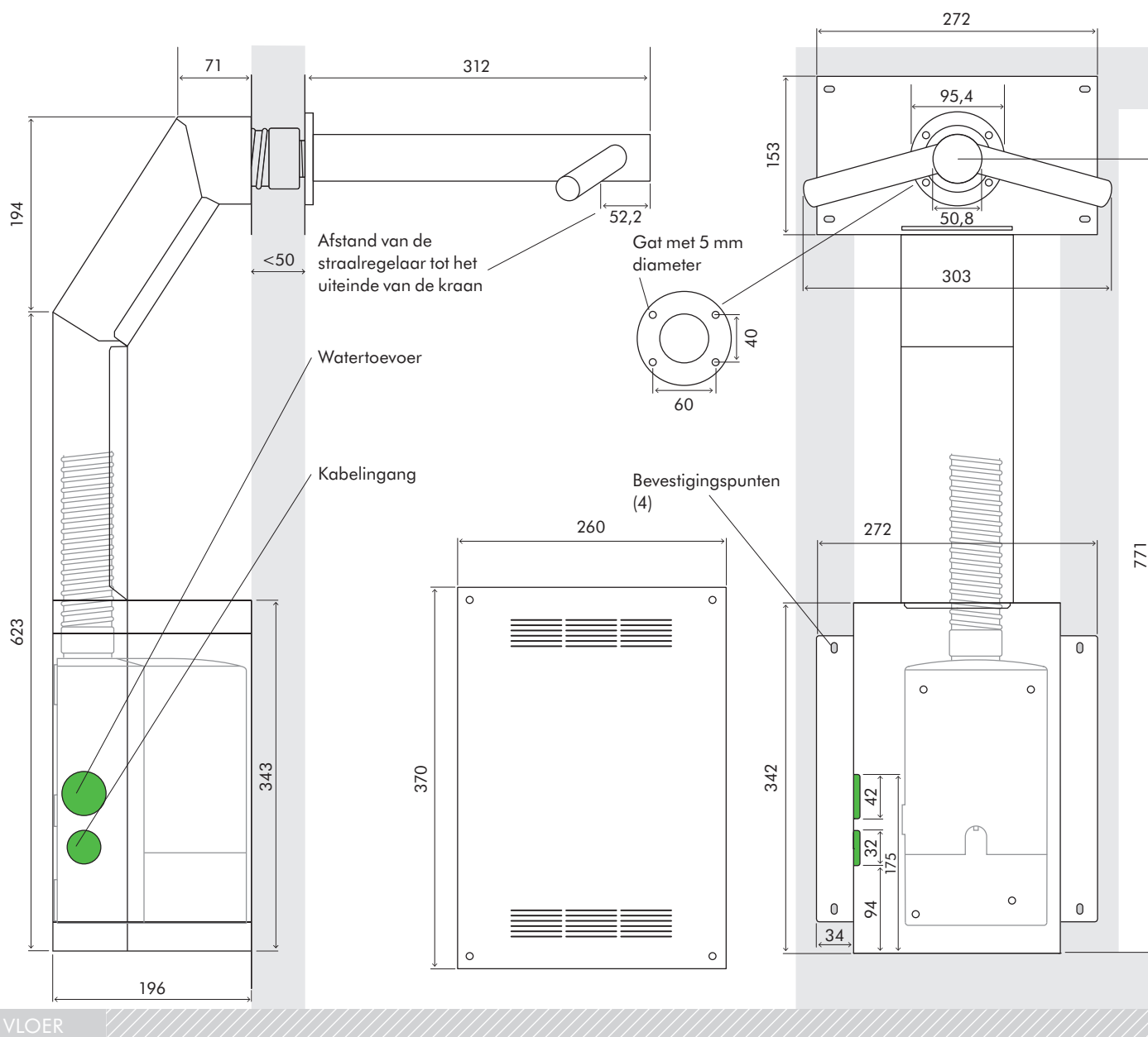
ZIJAANZICHT
