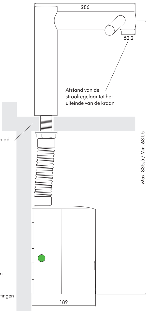
ZIJAANZICHT
