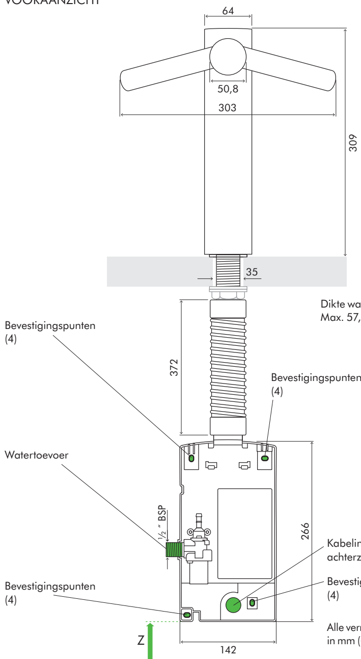
VOORAANZICHT
