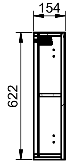
A-A ( 1 : 16 )
